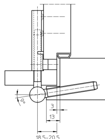
Querschnitt
