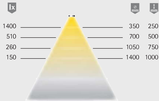
Lichtverteilungsdiagramm / 70° (Länge 600 mm)
